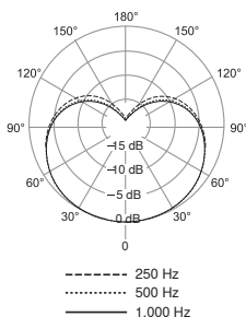
Диаграмма направленности
