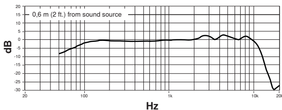
Амплитудно-частотная характеристика
