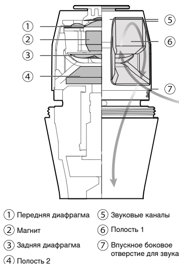
Картридж Dualdyne, вид сбоку
