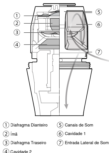
Vista lateral da cápsula do Dualdyne
